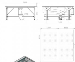
Electric Box Fan
